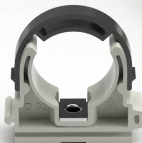
Příchytka s třmenem a kovovou maticí M6
